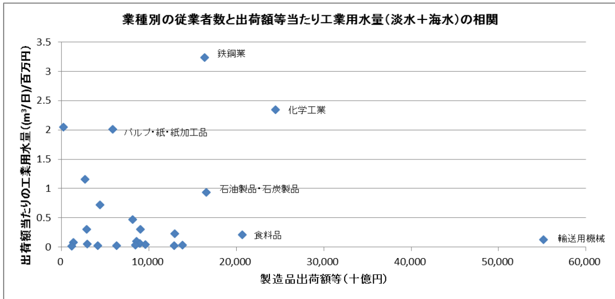
図2.1-8 平成24年度の製造品出荷額等当たりの用水量(淡水+海水)と従業者数の相関
